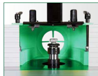
Frässpindel mit 80 mm Nutzlänge und 30 mm Durchmesser
