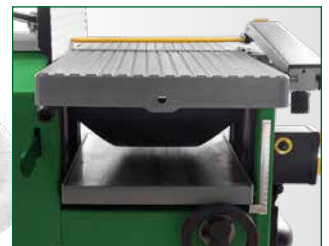
Dickenhobeln Höheneinstellung des Dickentisch einfach und bequem über Handrad und Skala Spanabnahme bis zu 2 mm möglich
