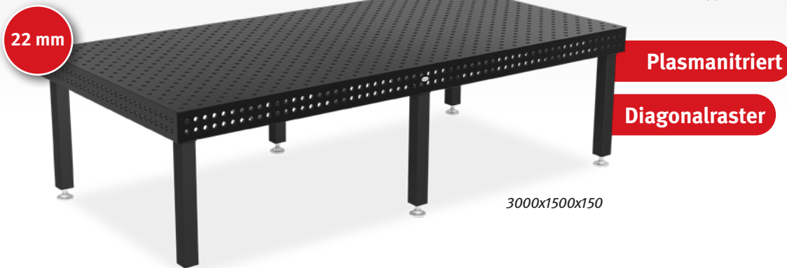
Schweißstisch Professional Extreme 8.7 aus durchgehärtetem Werkzeugstahl X8.7 plasmanitriert mit Diagonalraster
