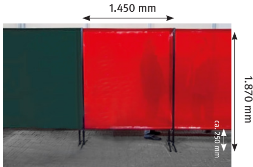
Abbildung zeigt mehrere Schutzwände aneinander gereiht
